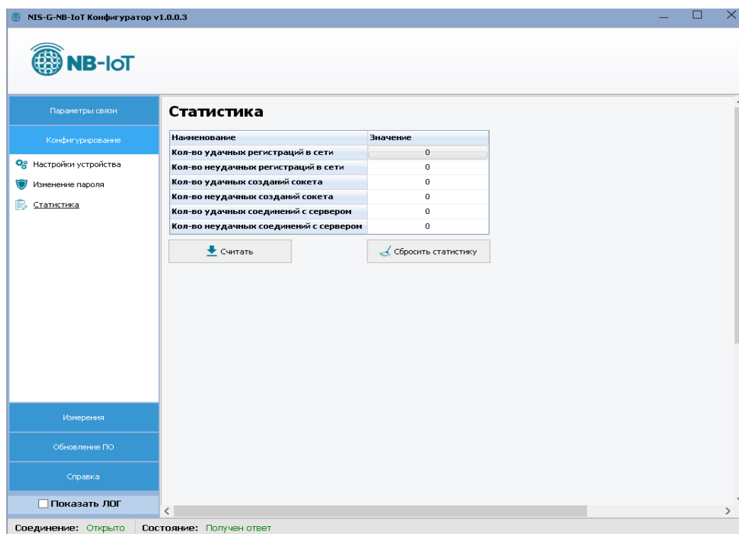
Рисунок 13 – Статистика
