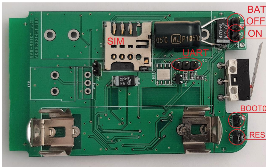
Рис. 2 – Вид платы и расположение интерфейсов.
